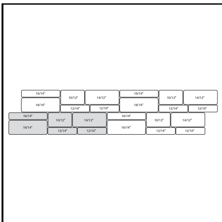
3" & 6" High 1:1 Module Ashlar
